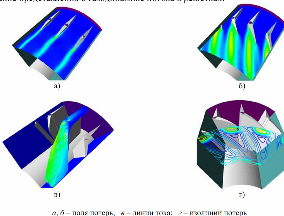
Рис. 3. Распределение потерь у периферии и в контрольном сечении
