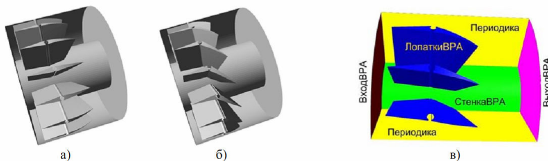
Рис. 2. Твердотельные модели ВРА при \theta = 0^\circ (а) и \theta = 45^\circ (б) и граничные условия (в) модели
