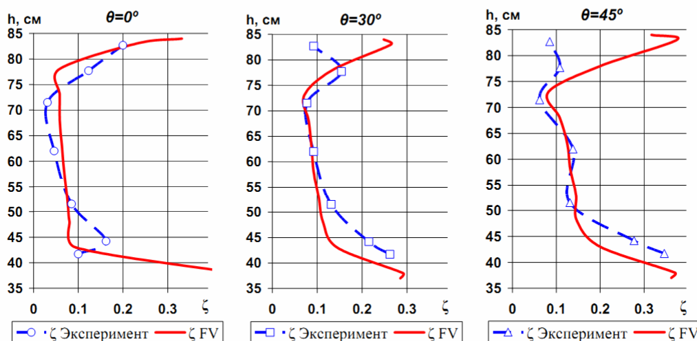
Рис. 5. Коэффициент потерь при разных углах поворота хвостовика
